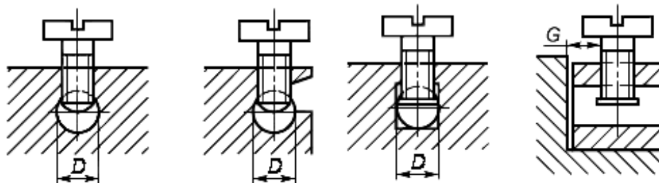
Контактные зажимы без прижимной пластины
