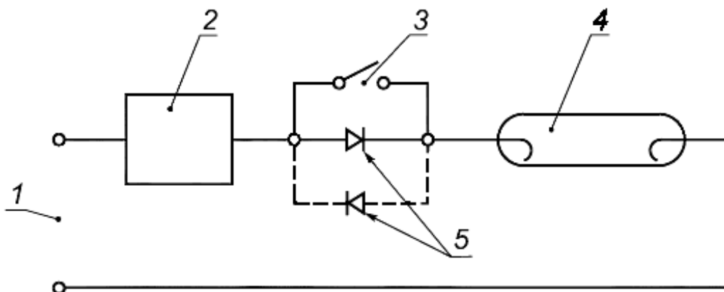
1 - сеть; 2 - испытуемый ПРА; 3 - выключатель; 4 - лампа; 5 - выпрямитель
