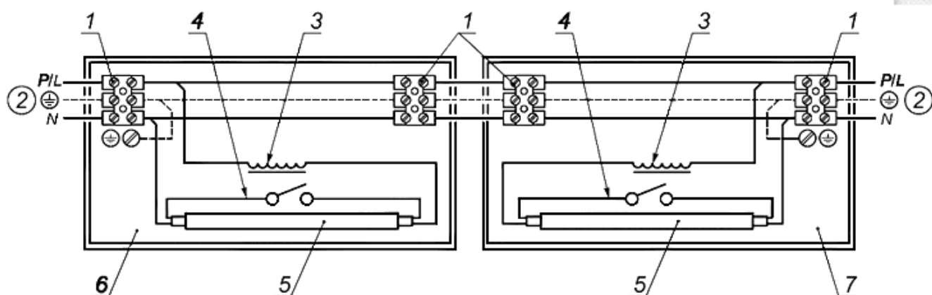
Рисунок 20А - Иллюстрация термина "шлейфовый способ присоединения"
