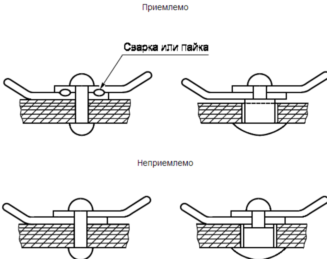
Рисунок 18 - Примеры безвинтовых контактных зажимов пружинного типа
