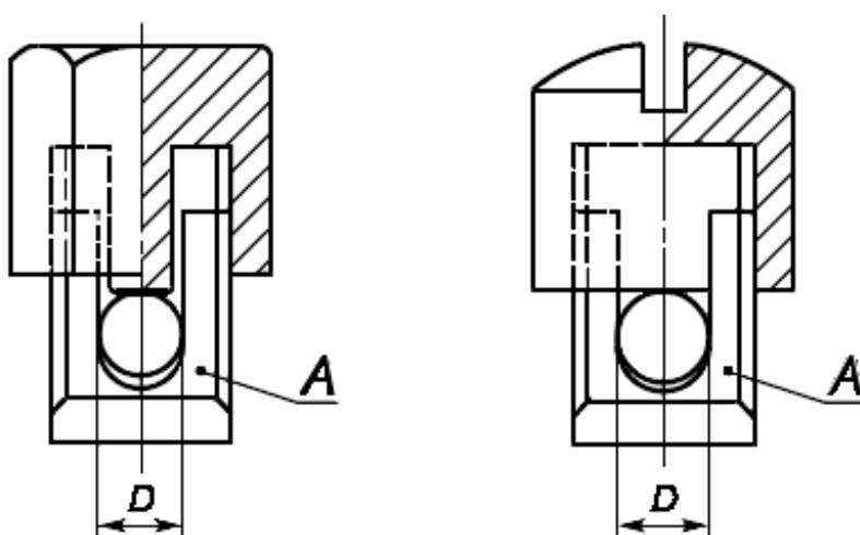
Рисунок 16 - Колпачковые контактные зажимы
