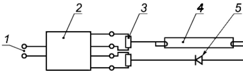
1 - сеть; 2 - испытуемый ПРА; 3 - резистор; 4 - лампа; 5 - выпрямитель
