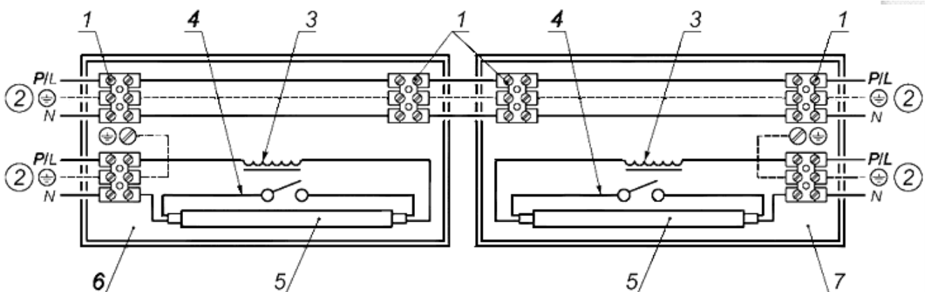
Рисунок 20В - Иллюстрация термина "сквозная проводка" с подключением светильника (может быть использовано для трехфазной сквозной проводки, когда подключение светильника чередуется между L1, L2, L3 и нейтралью)
