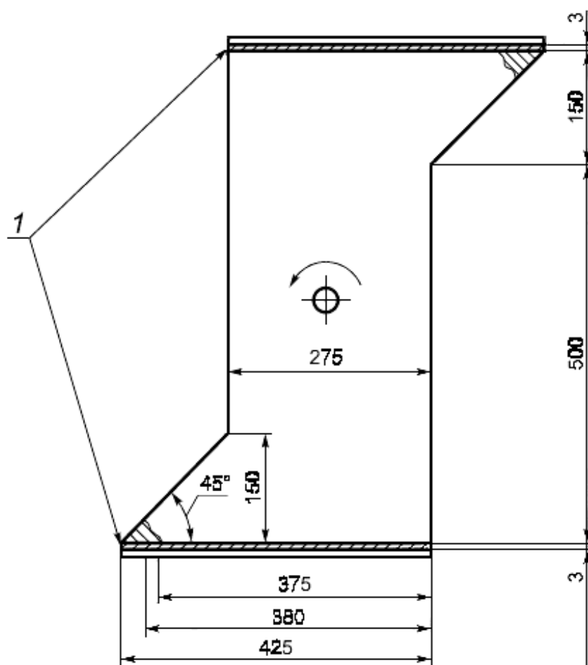
Рисунок 25 - Вращающийся барабан
