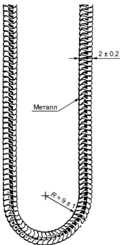
Рисунок 30 - Пример резьбоформирующего винта, используемого в пазу металлического материала
