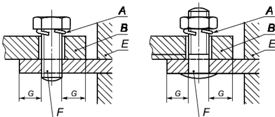
Рисунок 15 - Контактные зажимы для кабельных наконечников или плоских выводов
